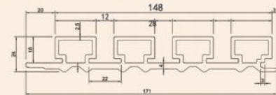
配套产品截面图 Products Sectional View Item: M1724 格栅
