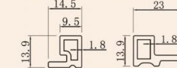
配套产品截面图 Products Sectional View Item: M148格栅收口
