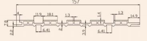
配套产品截面图 Products Sectional View Item: M159-2小长城
