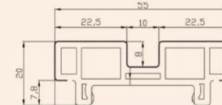
配套产品截面图 Products Sectional View Item: G55骨路线
