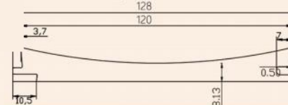
配套产品截面图 Products Sectional View Item: M128半圆板
