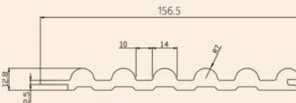
配套产品截面图 Products Sectional View Item: S156 半圆板
