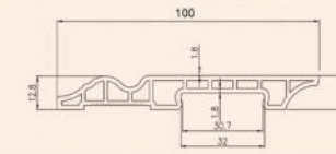
配套产品截面图 Products Sectional View Item: MT100 踢脚线
