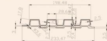
配套产品截面图 Products Sectional View Item: H2428大长城
