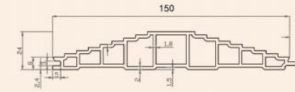
配套产品截面图 Products Sectional View Item: M150金字塔
