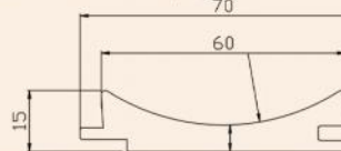
配套产品截面图 Products Sectional View Item: S7015-半月板
