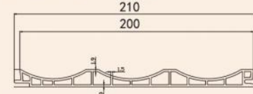
配套产品截面图 Products Sectional View Item: M210三圆板
