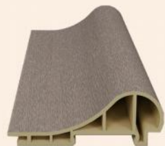
配套产品截面图 Products Sectional View Item: H80 小怀抱
