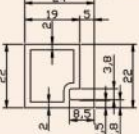
配套产品截面图 Products Sectional View Item: 170格栅收口B
