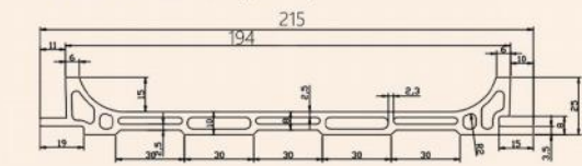
配套产品截面图 Products Sectional View Item: M2025玛格线
