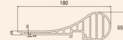
配套产品截面图 Products Sectional View Item: H180 转轴线
