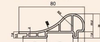
配套产品截面图 Products Sectional View Item: H80 小怀抱
