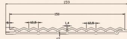
配套产品截面图 Products Sectional View Item: M159小三角板
