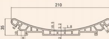
配套产品截面图 Products Sectional View Item: 2135 弓弦线
