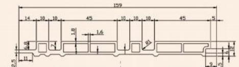
配套产品截面图 Products Sectional View Item: M1512格栅板
